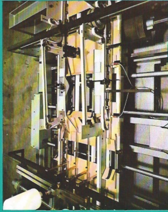
Dispositivo per la produzione di scatole con 4 angoli incollati a richiesta
