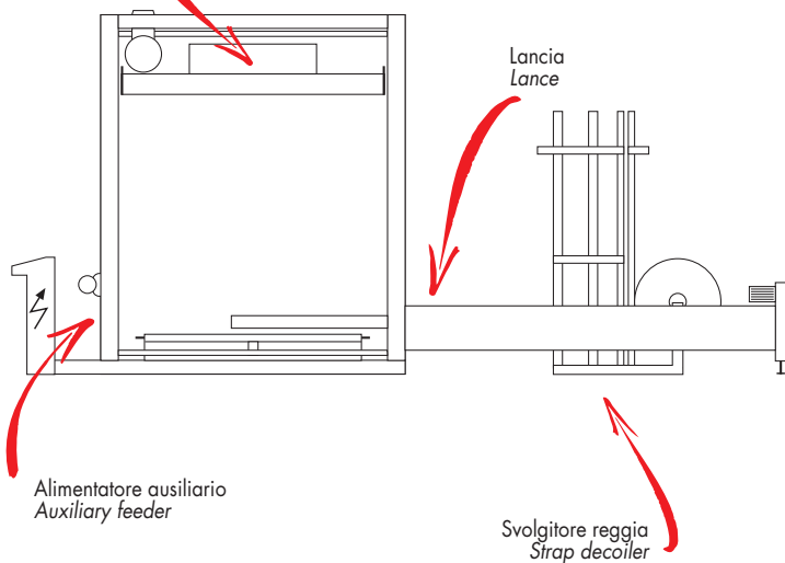
Testata reggiante Strapping head
